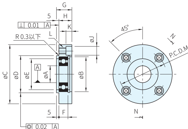
斷面 N-N
